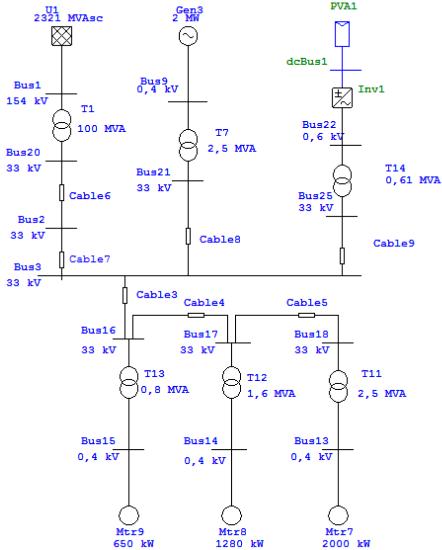
Şekil 3. Fabrikaya ait tek hat şeması
