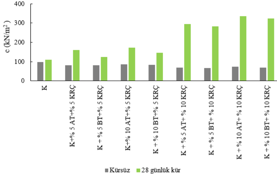
Şekil 10. İki Katkı Malzemesi Kullanılan Örnekler Ait Kür Öncesi ve Kür Sonrası c Değerlerini Gösteren Histogram
