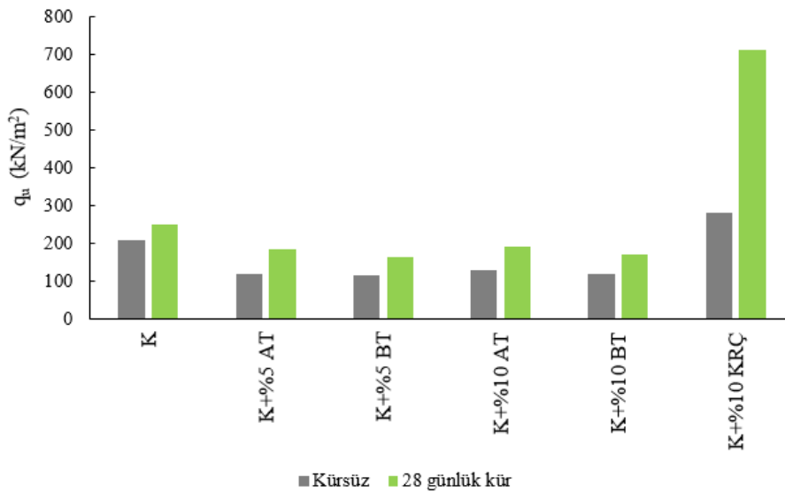
Şekil 7. Tek Katkı Malzemesi Kullanılan Örneklerin Kür Öncesi ve Kür Sonrası q_u Değerlerini Gösteren Histogram
