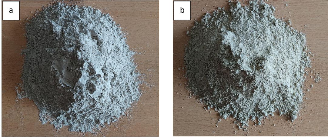
Şekil 2. a. Çalışmada Kullanılan Asidik Tüf b. Bazik Tüf
